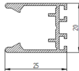
profilé latéral en aluminium de 25mm
