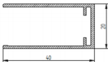
canal aimanté
